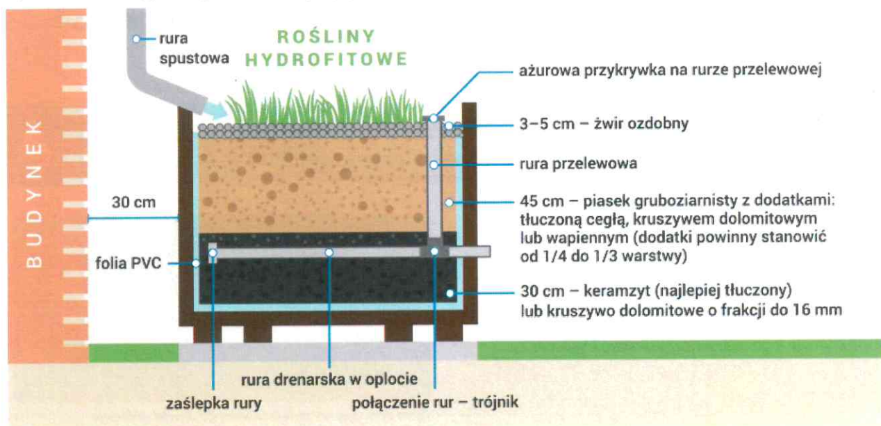
Rysunek 2. Przekrój przez ogród deszczowy w pojemniku
